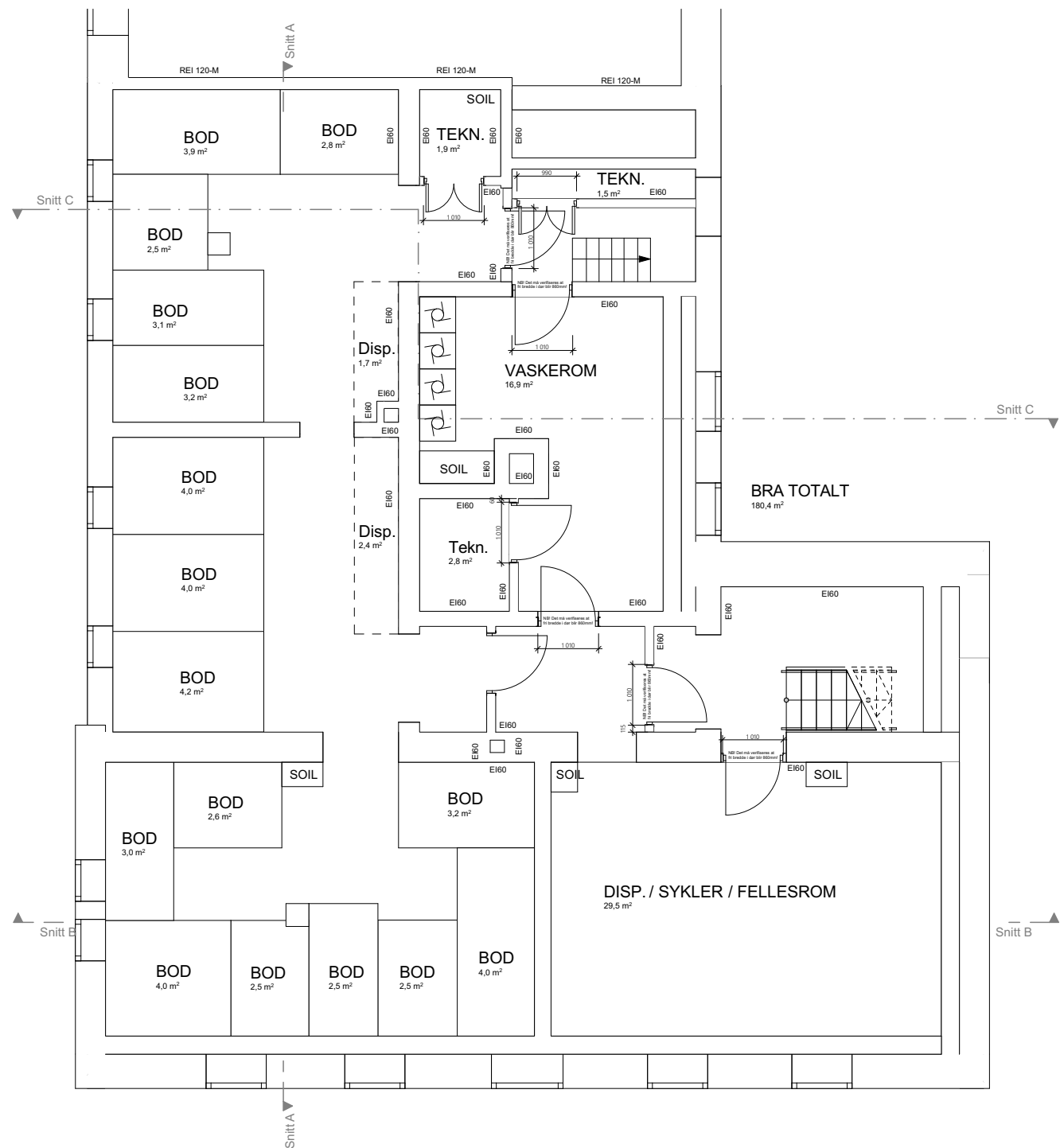
U.Etasje 1:100
